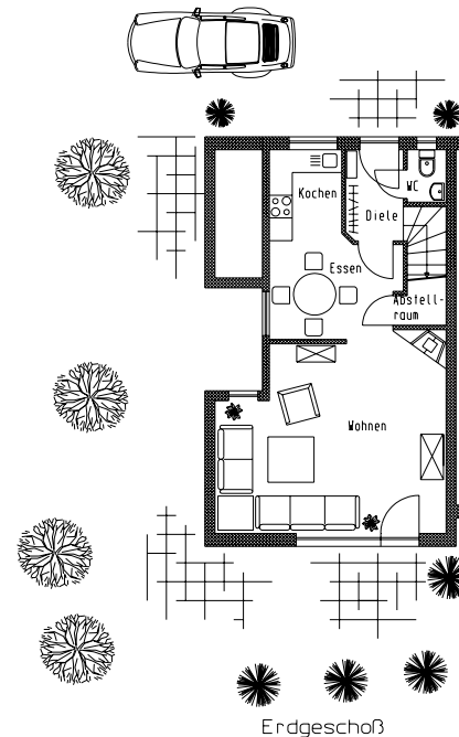
Erdgeschoß
